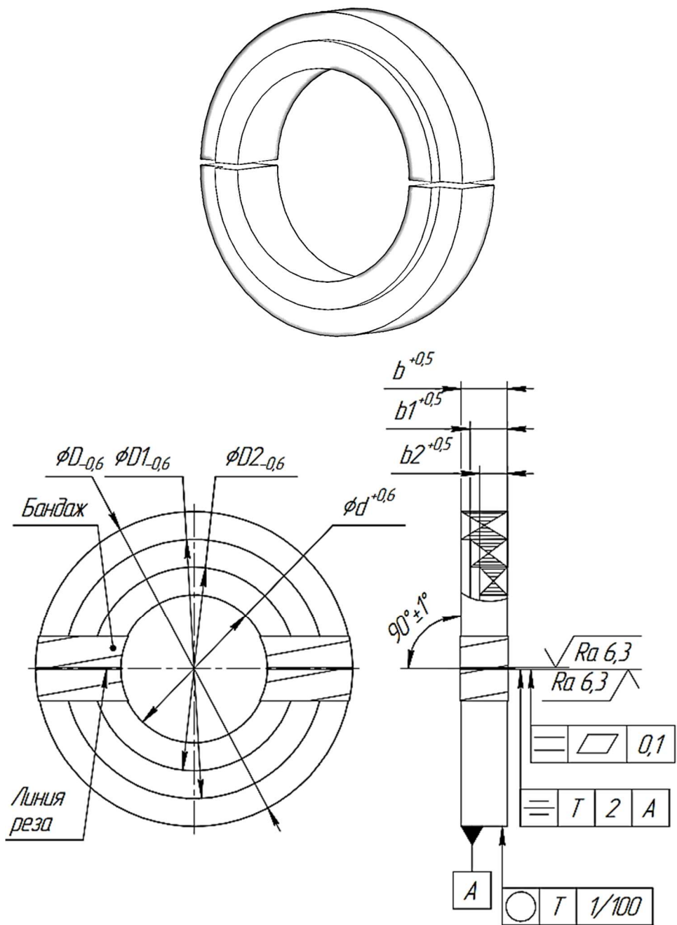
Рис. Б10. Размеры магнитопровода ОЛСР
