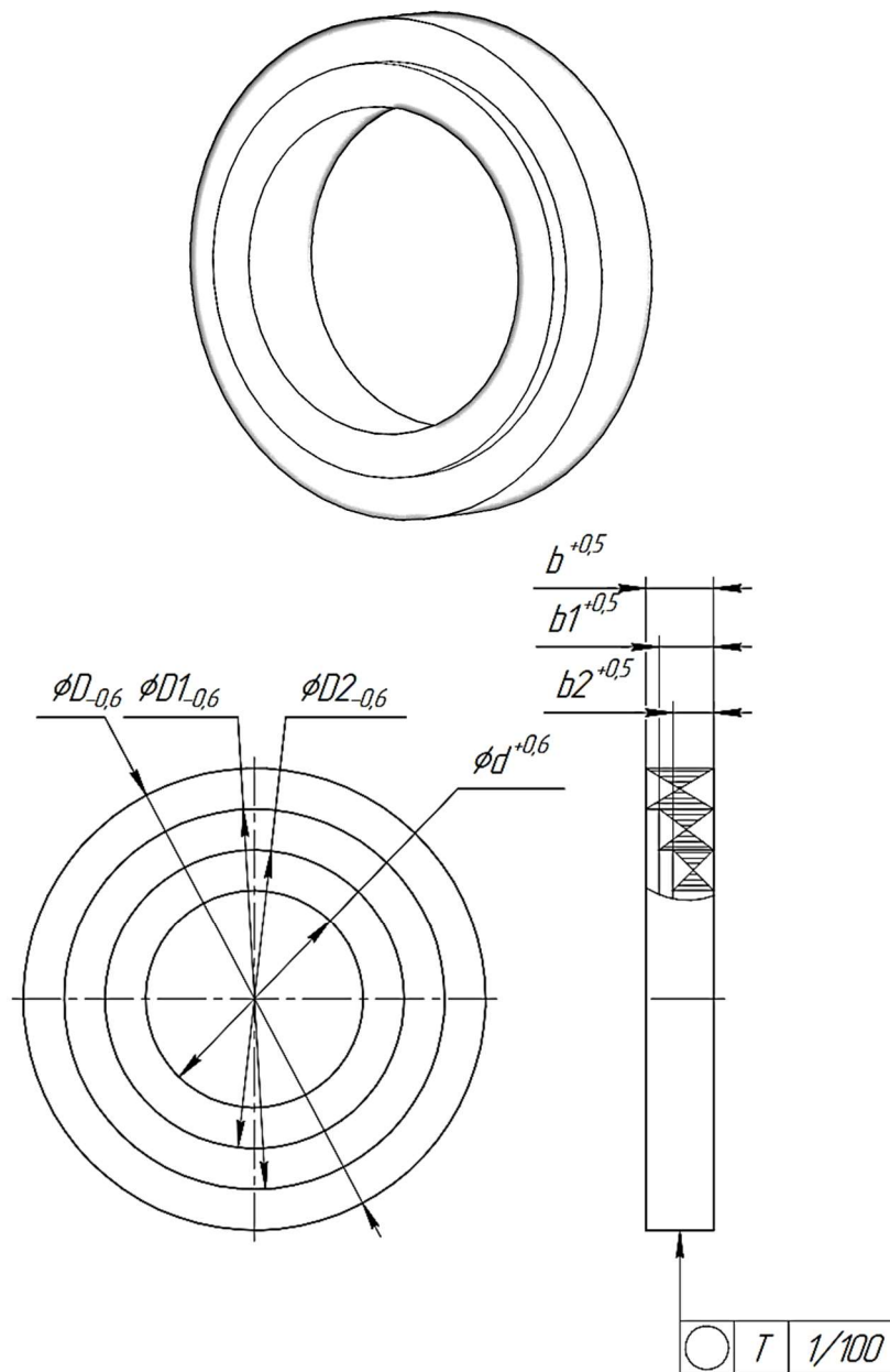
Рис. Б9. Размеры магнитопровода ОЛС
