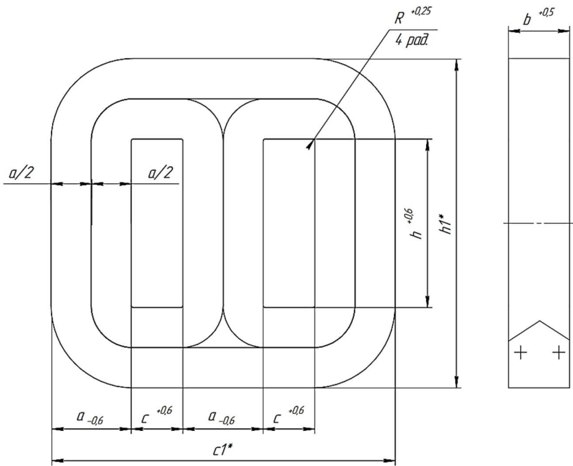
Рис. Б6. Размеры магнитопровода ТЛ
