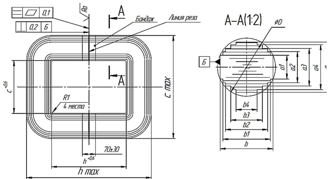
Рис. Б12. Размеры магнитопровода ПЛСР
