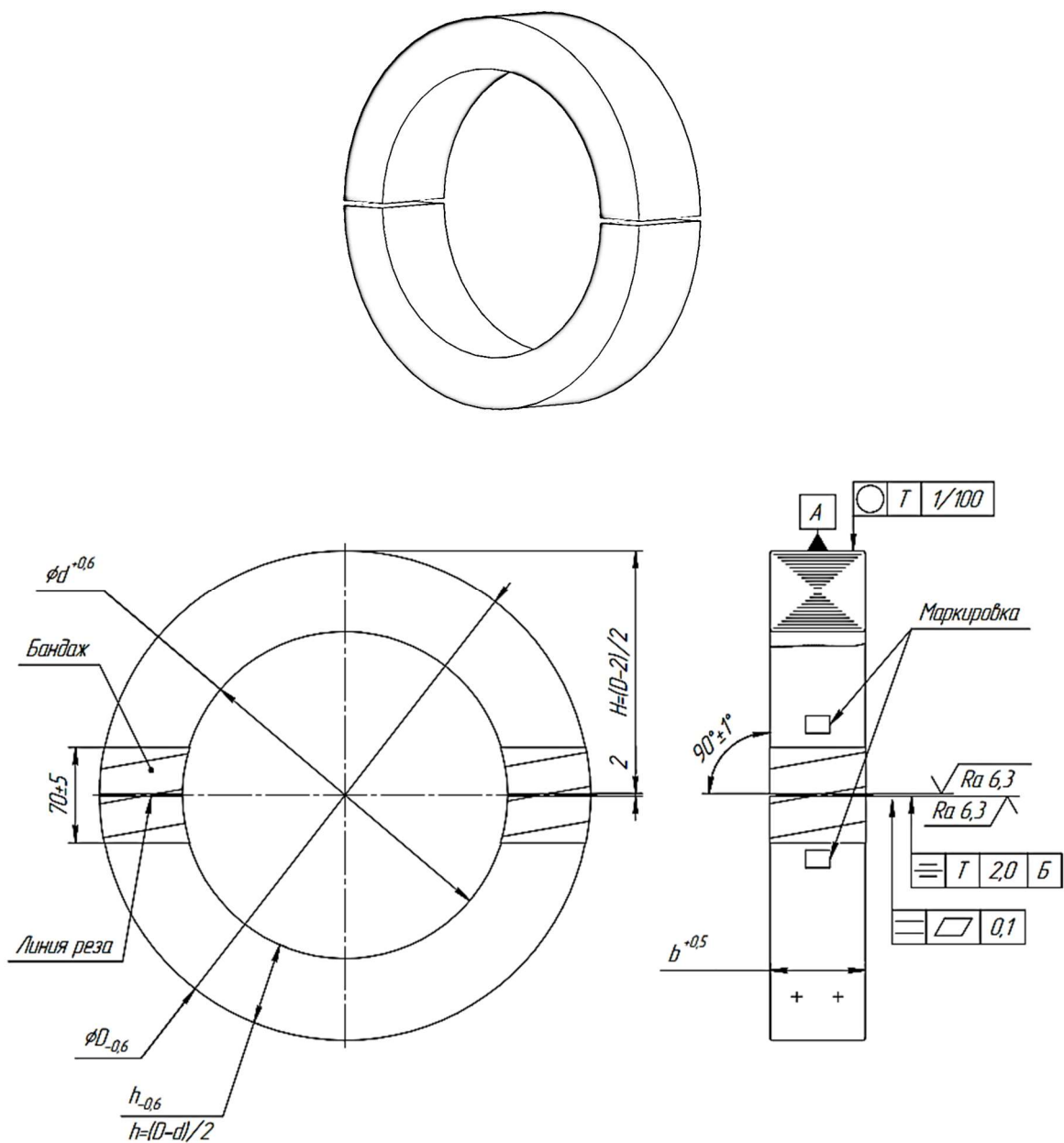
Рис. Б2. Размеры магнитопровода ОЛР
