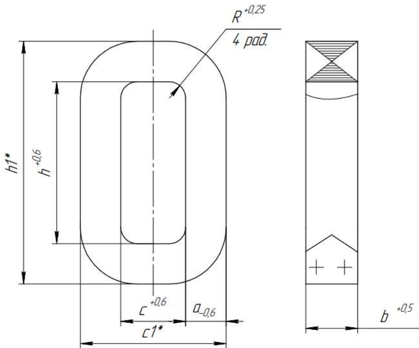
Рис. Б3. Размеры магнитопровода ПЛ
