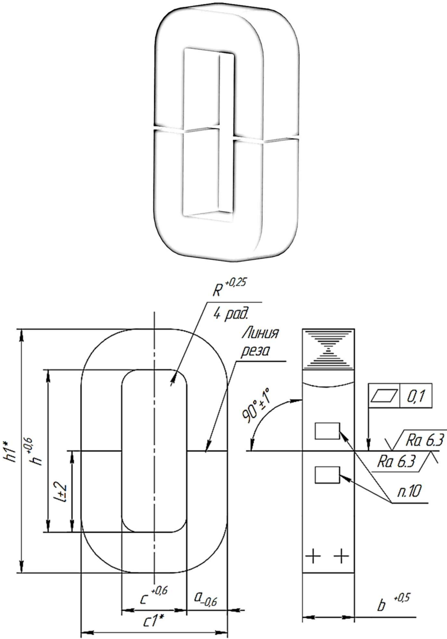
Рис. Б4. Размеры магнитопровода ПЛР
