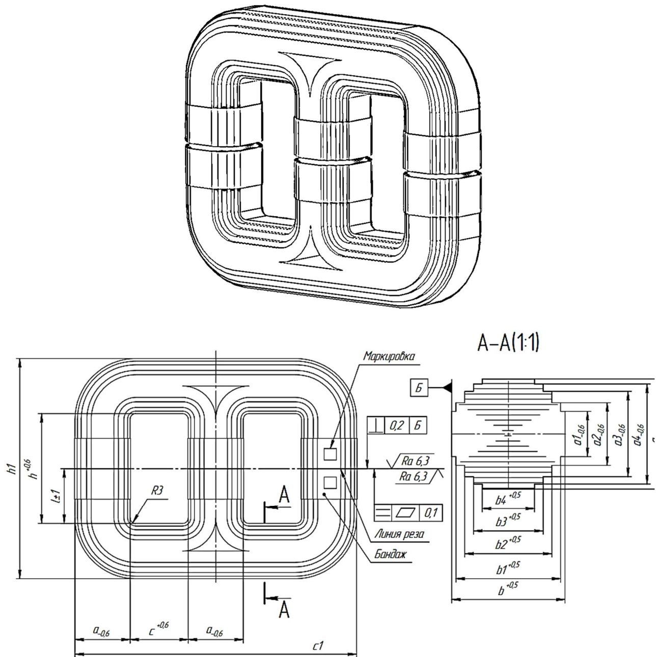
Рис. Б14. Размеры магнитопровода ТЛСР
