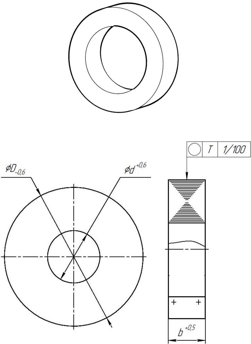
Рис. Б1. Размеры магнитопровода ОЛ
