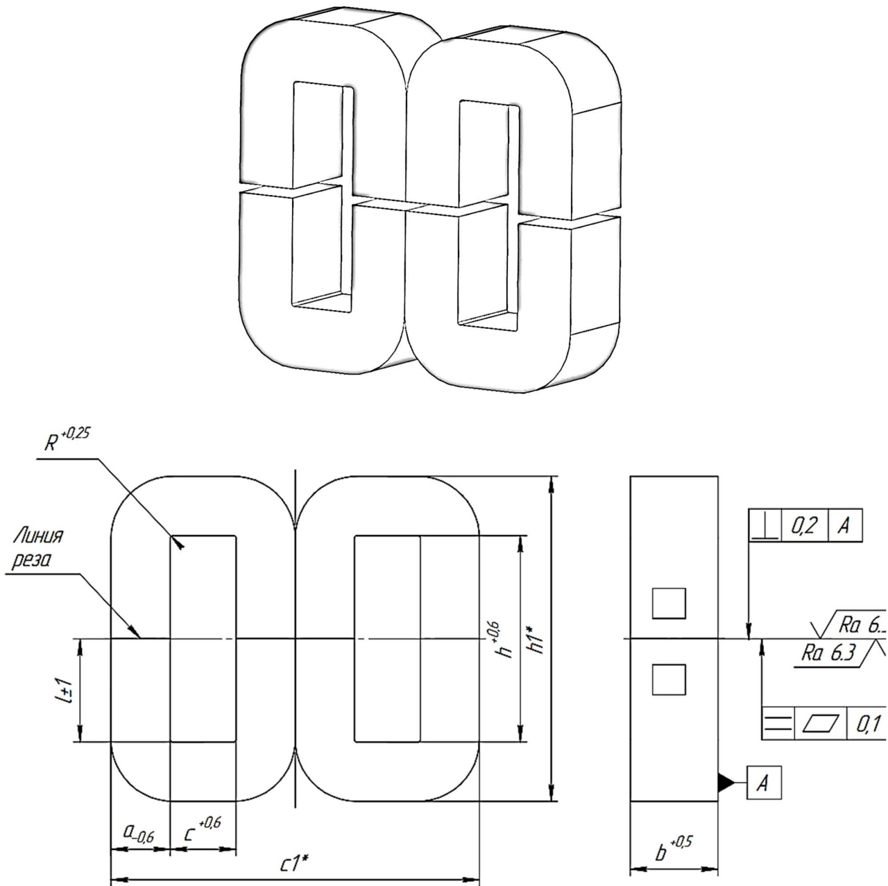
Рис. Б7. Размеры магнитопровода ШЛР
