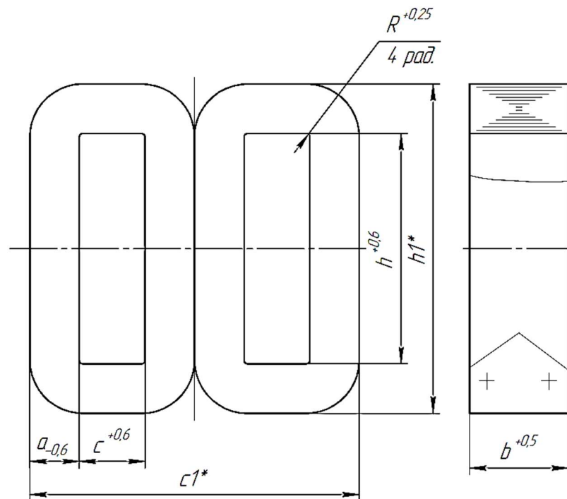
Рис. Б5. Размеры магнитопровода ШЛ
