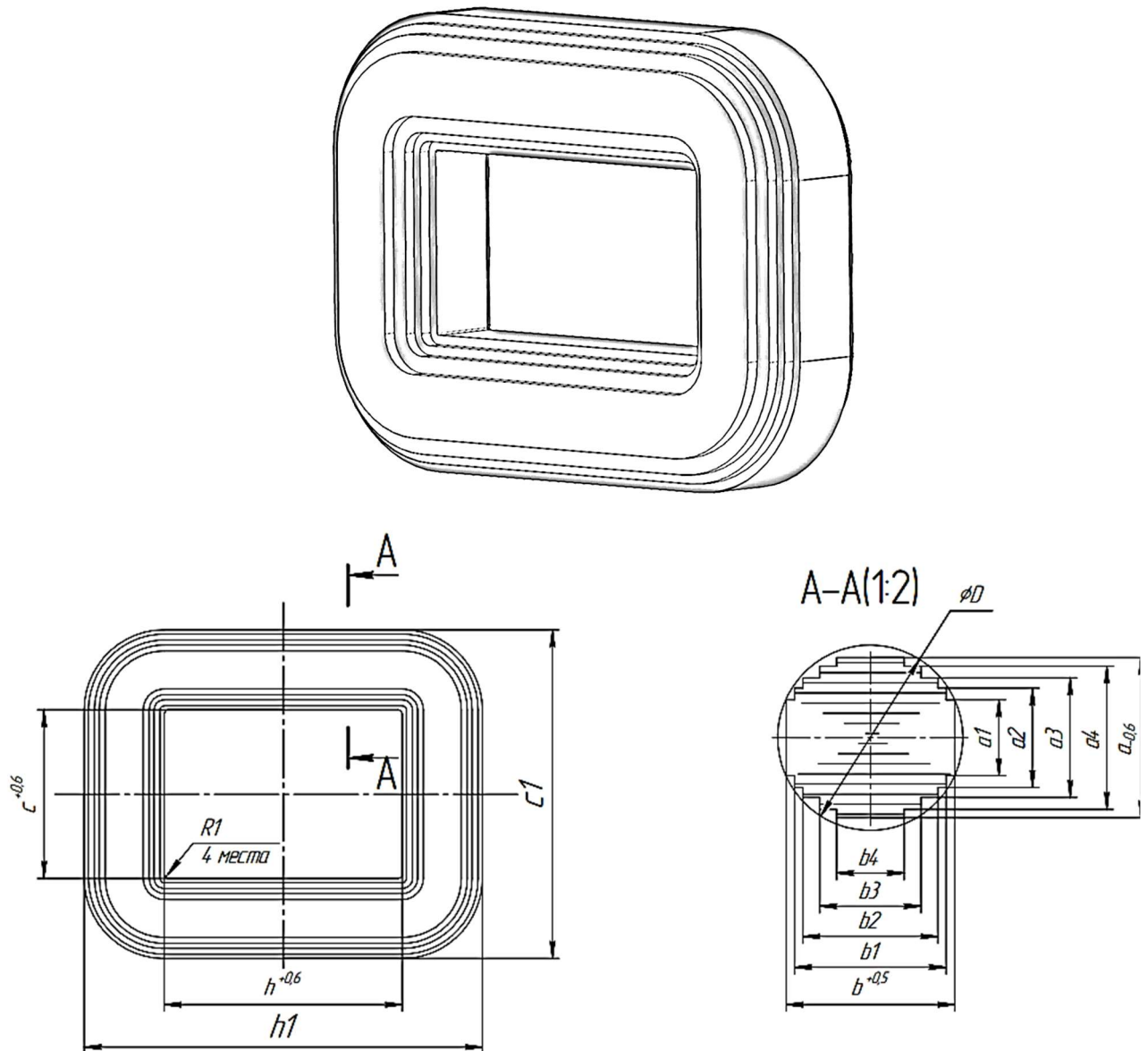
Рис. Б11. Размеры магнитопровода ПЛС
