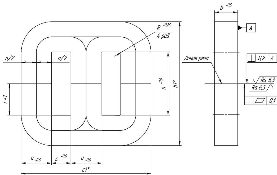
Рис. Б8. Размеры магнитопровода ТЛР Структура условного обозначения магнитопровода ТЛР
