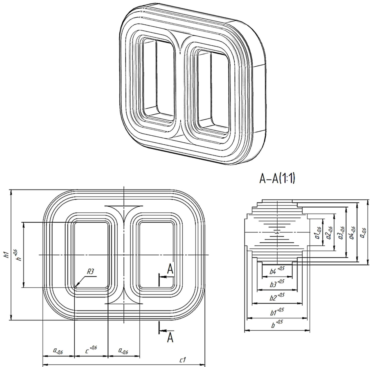
Рис. Б13. Размеры магнитопровода ТЛС
